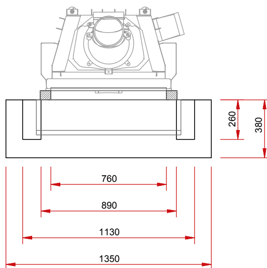
Изображение сверху М 1:25
